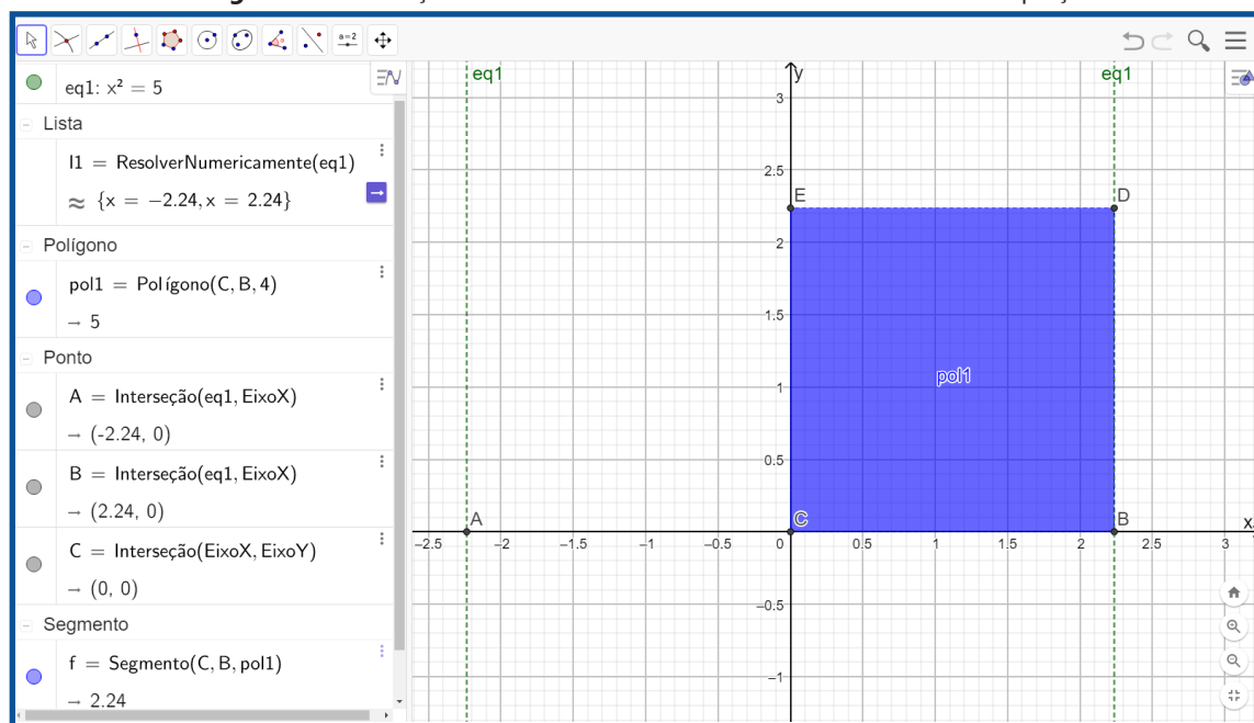
Figura 50: Resolução com o comando "Resolver Numericamente" a equação.
